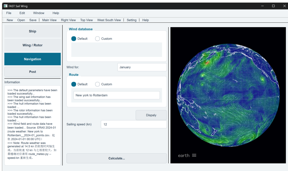
图 9 航线气象模块界面
