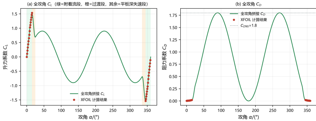
图 3 全攻角极线的三段式拼接结果
