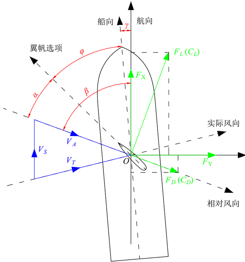
图 1 风翼受力简图 ( \beta 、 \alpha 、 \varphi 为本文所用角度体系)
