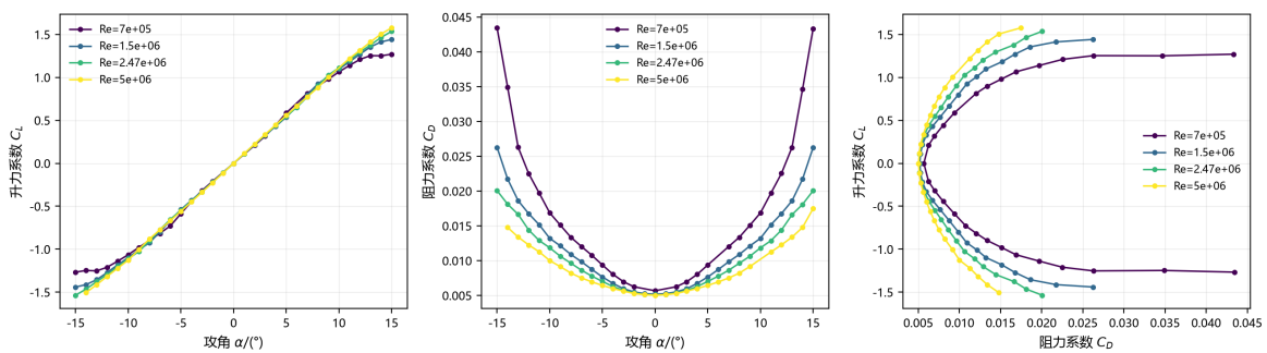
图 2 翼帆翼型极线的 XFOIL 计算结果
