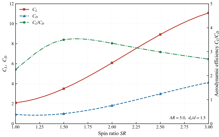
图 4 转筒帆升阻力系数与气动效率随转筒比的变化 ( AR = 5.0 , d_e/d = 1.5 )
