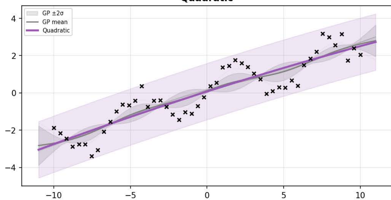
Quadratic
