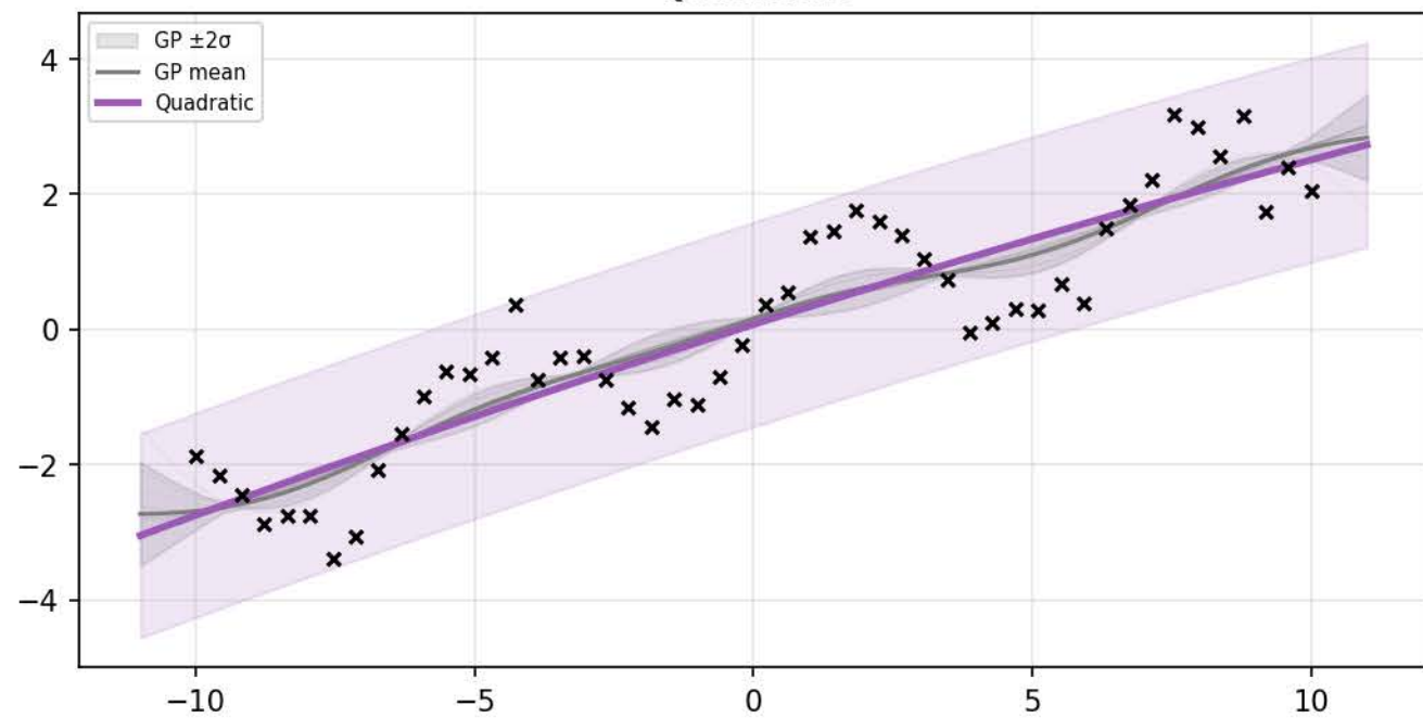
Quadratic
