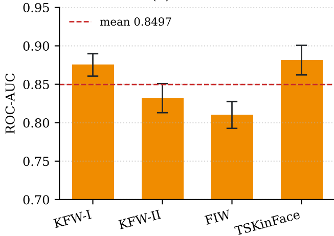
(b) ROC-AUC
