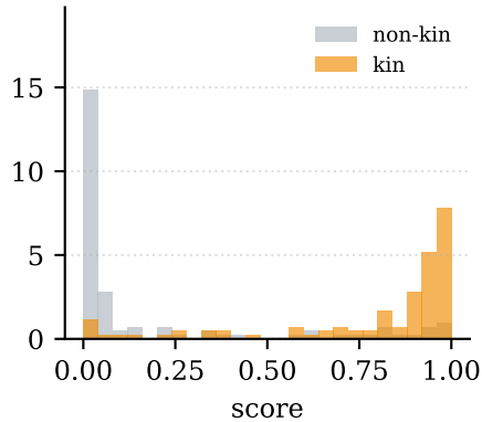
KFW-I
