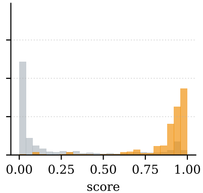
TSKinFace
