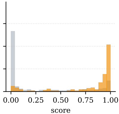
KFW-II
