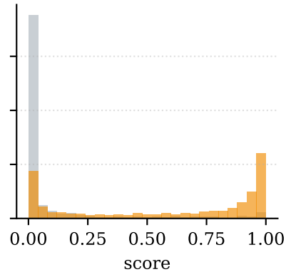
FIW
