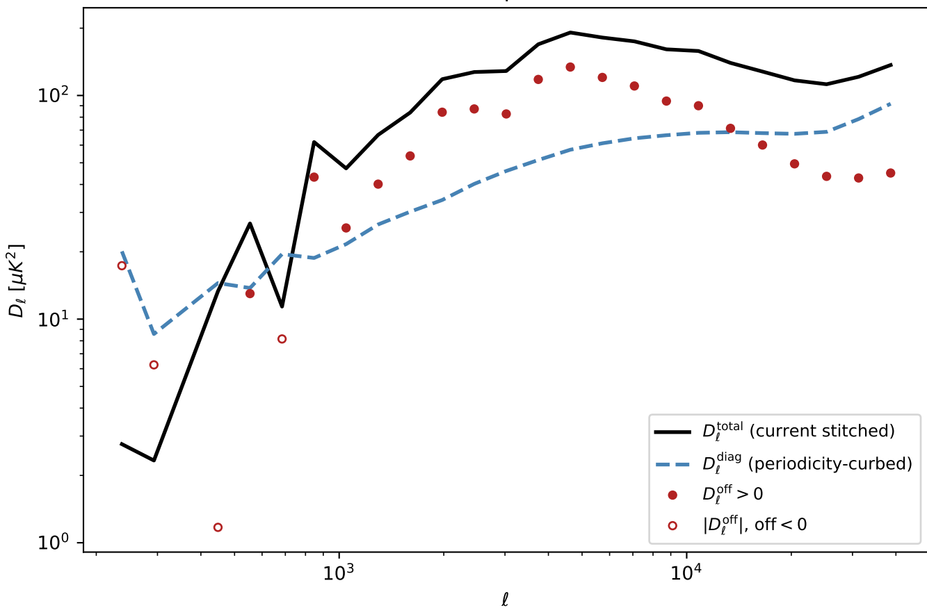
kSZ auto-power coherence decomposition -- seed 1 (300 Mpc box)
