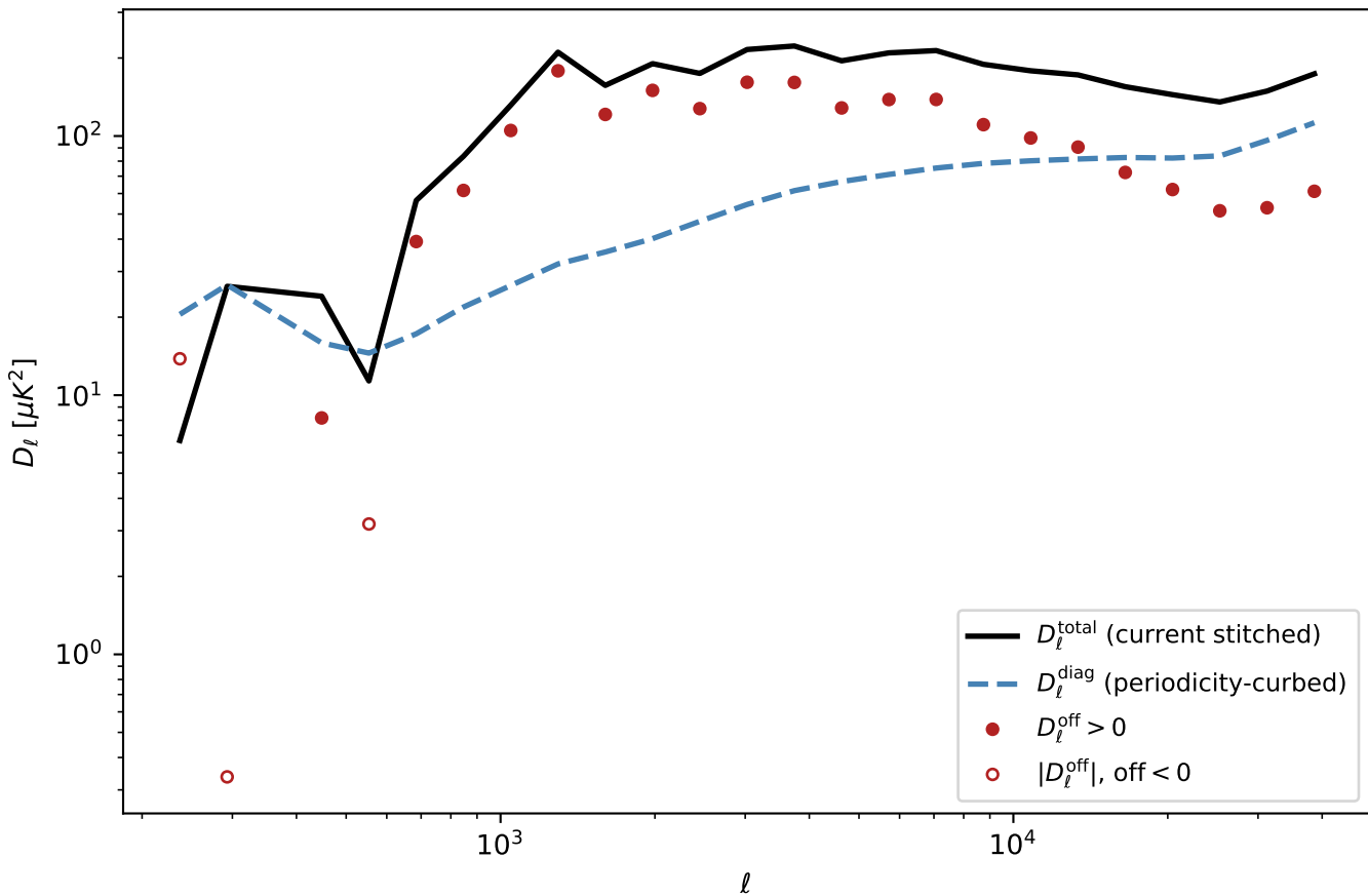
kSZ auto-power coherence decomposition -- seed 3 (300 Mpc box)
