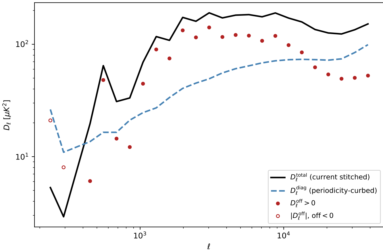
kSZ auto-power coherence decomposition -- seed 9 (300 Mpc box)
