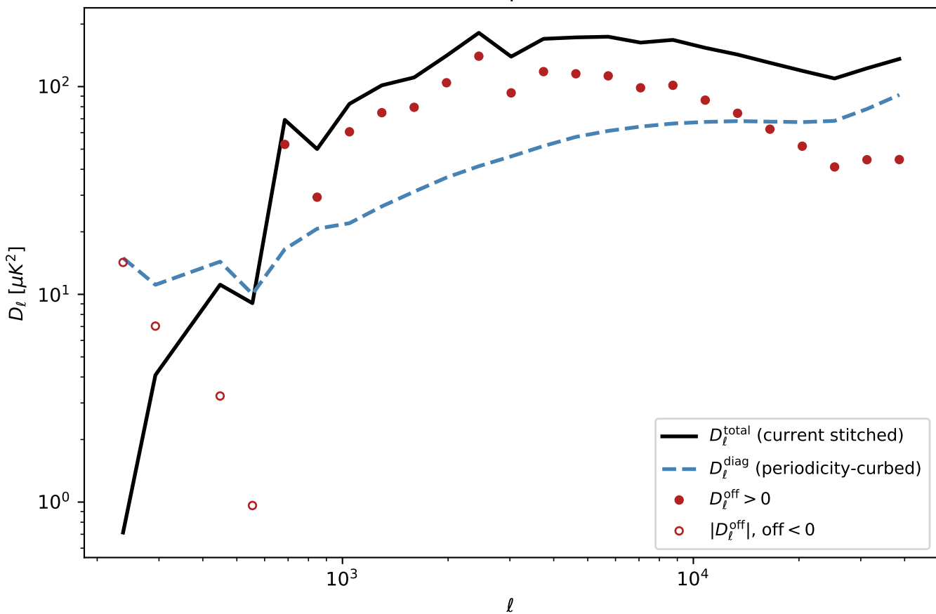
kSZ auto-power coherence decomposition -- seed 2 (300 Mpc box)
