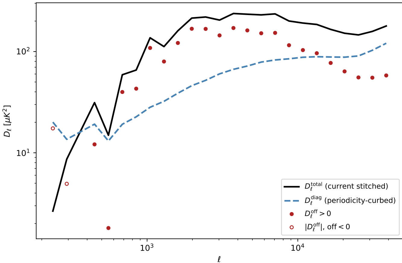
kSZ auto-power coherence decomposition -- seed 5 (300 Mpc box)
