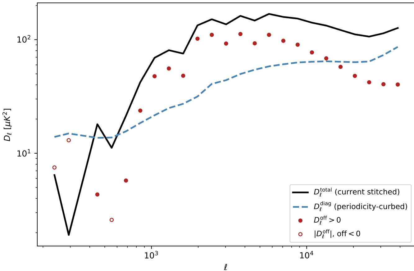
kSZ auto-power coherence decomposition -- seed 7 (300 Mpc box)
