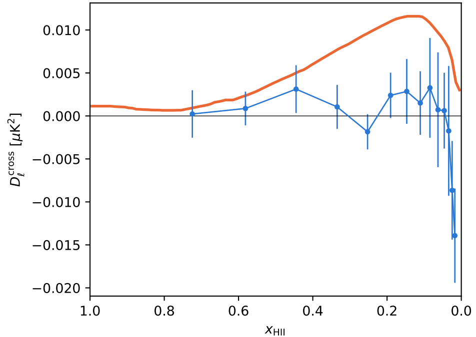
\ell = 3000 (SO)
