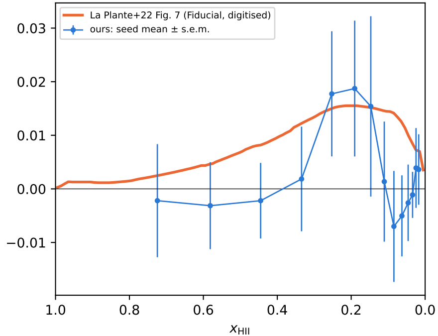
\ell = 500 (SO)
