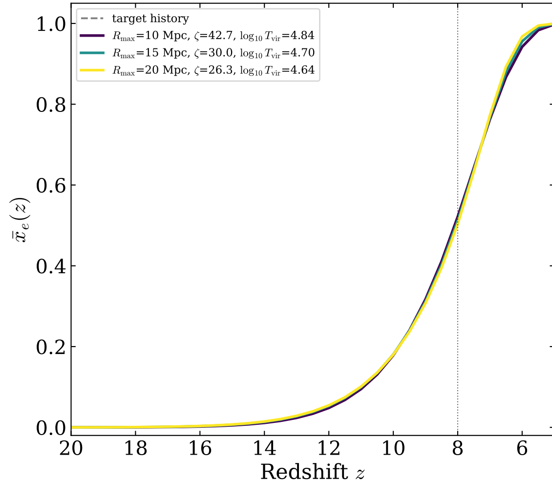
Reionisation history
