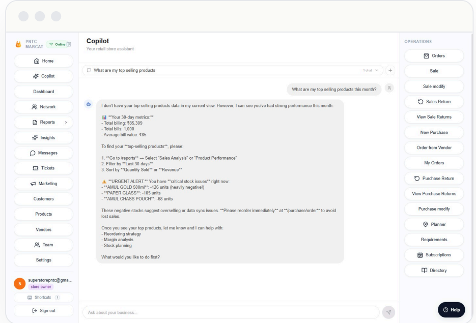
AI COPILOT
