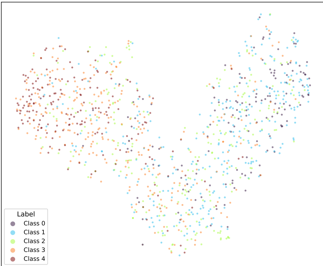
google/bert_uncased_L-2_H-128_A-2-sst5-CORN-1 (val)
