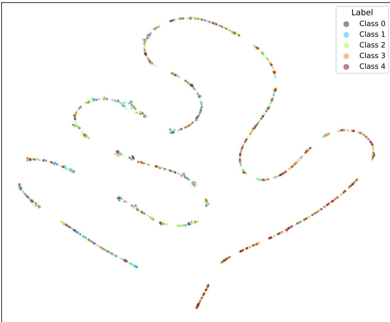
google/bert_uncased_L-2_H-128_A-2-sst5-CORN-2 (val)
