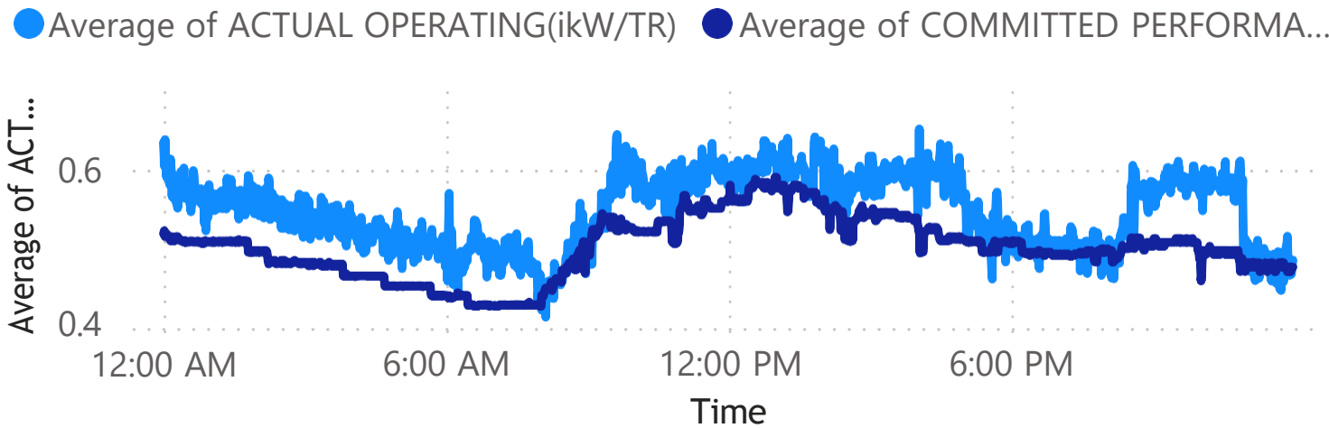
ACTUAL V/S COMMITED IKW/TR
