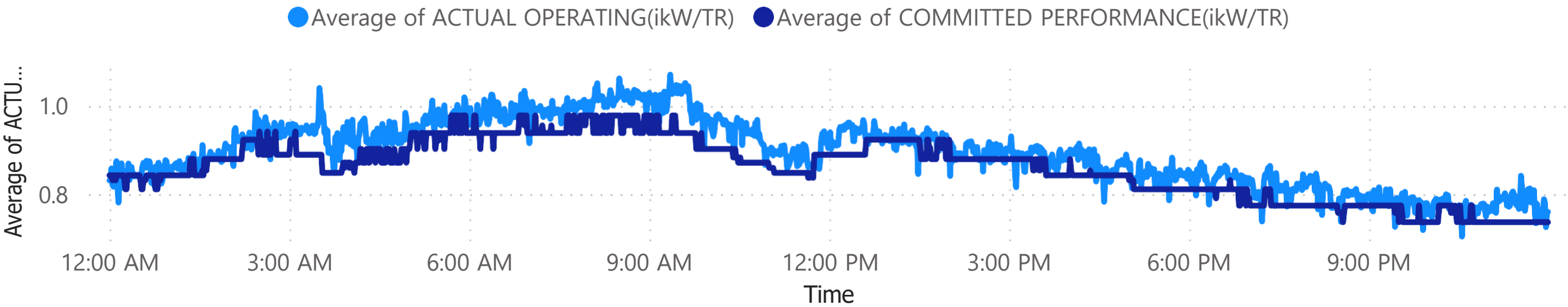
ACTUAL (kW/TR) V/S COMMITTED (ikW/TR)
