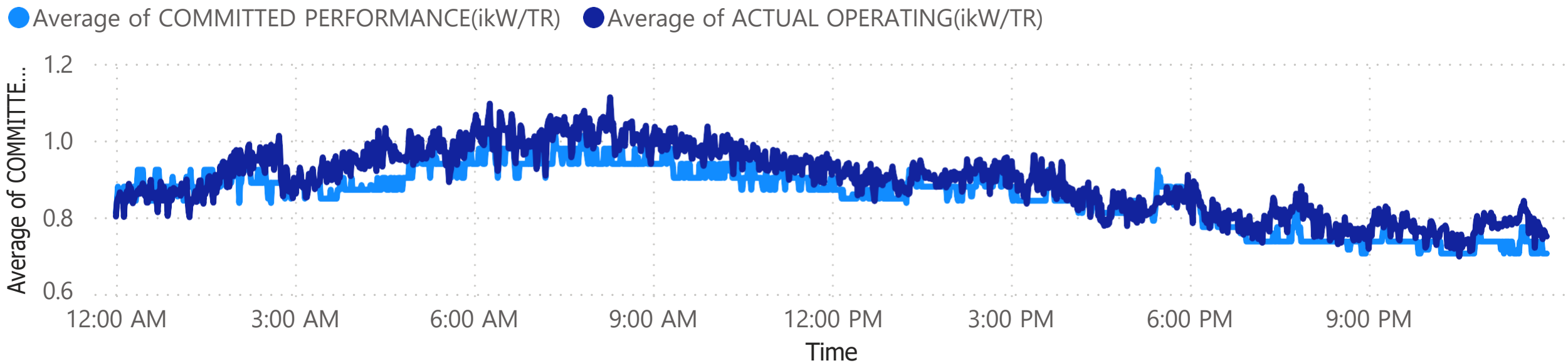
ACTUAL (kW/TR) V/S COMMITTED (ikW/TR)
