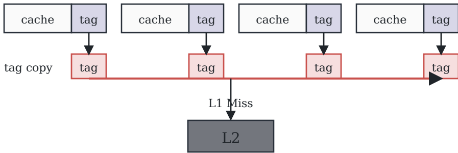
(d) RING [16] cache sharing
