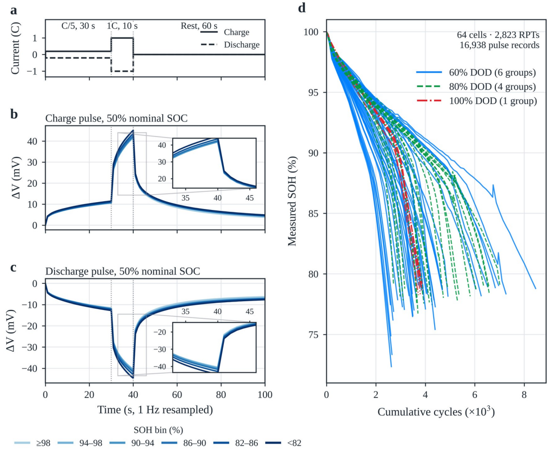
图 1 数据集与脉冲响应。(a) 充电（实线）与放电（虚线）脉冲的程控电流：C/5 电流 30 s、1C 电流 10 s、静置 60 s。(b, c) 50%名义 SOC 下相对脉冲前电压的平均电压响应 \Delta V ，按实测 SOH 分组（颜色越深表示 SOH 越低）；插图放大了 1C 段末端与弛豫起始处，该处过电位随老化增大。(d) 64 个电芯的实测 SOH 随累计循环数的变化，按放电深度着色；折线连接实测 RPT，不作插值。
