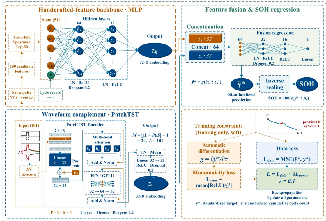
图 2 双分支 SOH 估计模型（R0 配置）。左上：人工特征主干；训练折筛选的 50 项特征与标准化累计循环数 \tau 组成 51 维输入，经 MLP 编码为 32 维表征。左下：波形补充；101 点脉冲电压响应经首点作差与逐位置标准化后，划分为 24 个片段（片段长度 P=9 ，步长 S=4 ），由单层 PatchTST 编码为 32 维表征。右：两路表征拼接为 64 维，经回归得到标准化 SOH \hat{y}^* ，再经逆标准化输出。训练最小化均方误差与正偏导 \partial \hat{y}^*/\partial \tau 惩罚项之和（ \lambda=0.1 ）；该软约束仅在训练中起作用。
