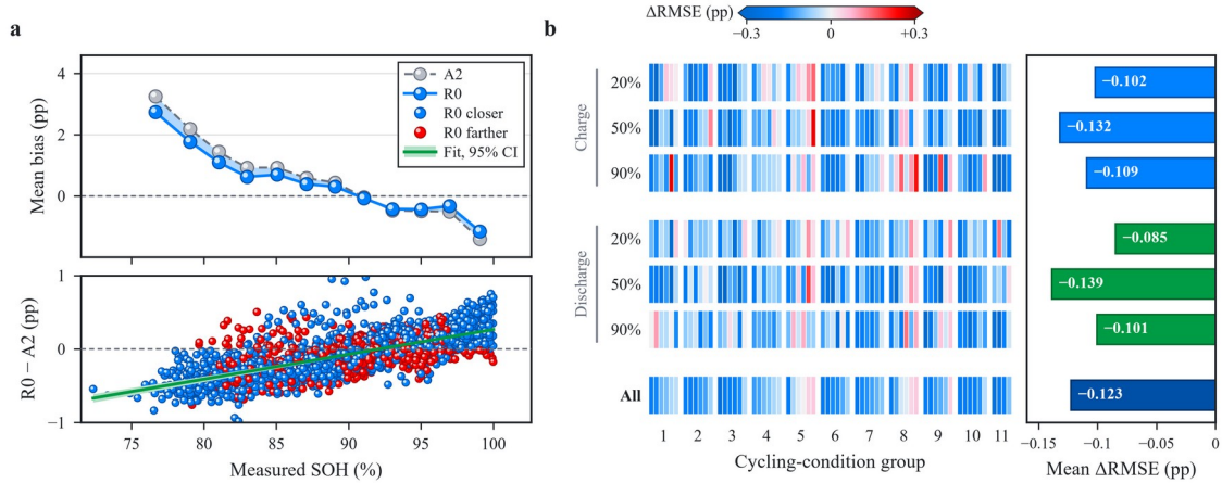
图 5 波形补充对偏差的修正及其在工况与电芯间的分布。(a) 上：按实测 SOH 每 2 个百分点分箱（低于 78% 的箱合并）的平均偏差（预测减真实值），灰色为 A2，蓝色为 R0；阴影表示被修正的偏差。下：2,823 个电芯-RPT 点上 R0 - A2 的预测改变量（蓝色表示更接近实测值，红色表示更远离），以及最小二乘拟合及其 95% bootstrap 区间带。预测均对种子和工况取平均。(b) 左：六个工况及全部记录上的逐电芯 R0 - A2 RMSE 差（电芯按循环工况组排列；超出 \pm 0.3 个百分点者颜色饱和）。右：各行的电芯宏平均差；所有 95% 区间均不含零。
