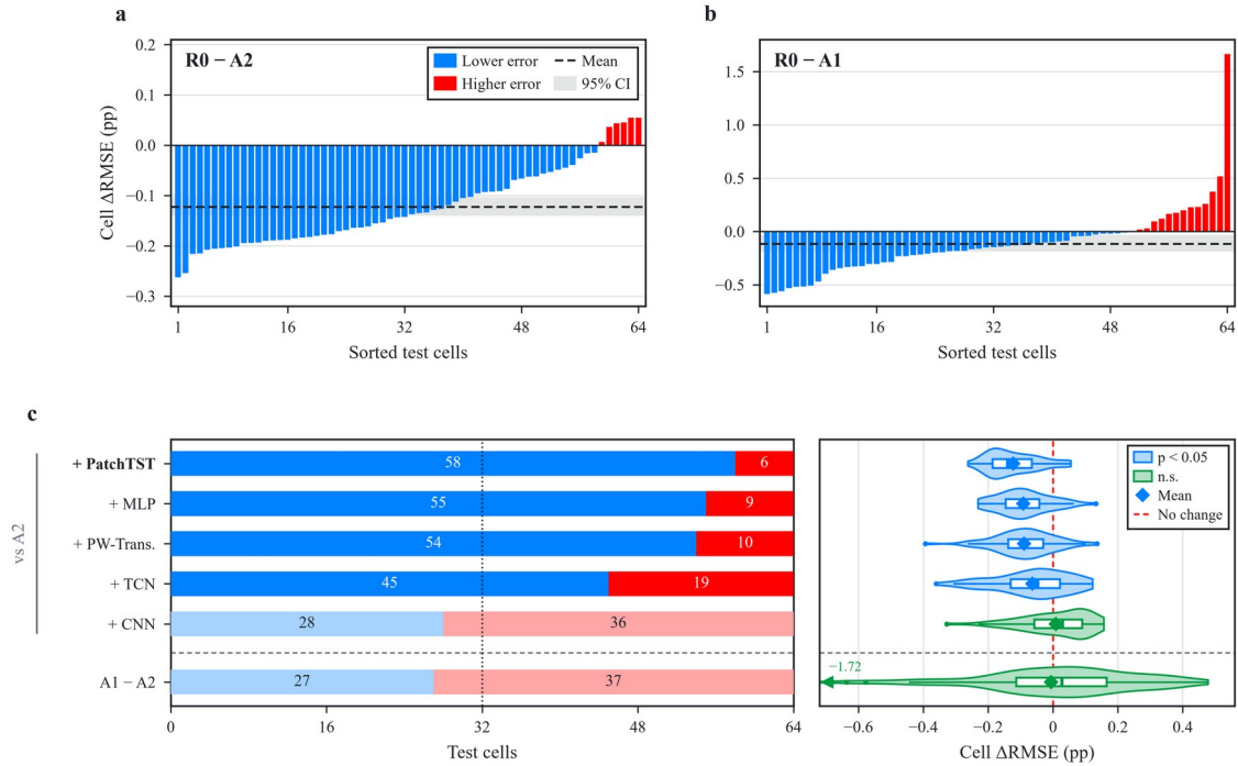
图4 人工特征主干与波形补充的作用。(a) 64 个测试电芯的逐电芯 RMSE 差 R0 - A2 (种子平均)，按升序排列；蓝色柱表示 R0 误差更低，红色柱表示更高；虚线与灰带为平均差及其 95% 区间。(b) 同(a)，为 R0 - A1；最右侧一柱为电芯 3。(c) 左：MLP 主干加入各补充后误差降低 (蓝) 或升高 (红) 的电芯数，以及 A1 相对 A2 的情况 (虚线下方)；浅色表示差异不显著。右：64 个配对差的小提琴图与箱线图 (箱体为四分位距，线为中位数，须线延伸至 1.5 倍四分位距，菱形为均值)；超出坐标范围的一个值 (A1 - A2, -1.72 个百分点，电芯 3) 标于左侧边缘。
