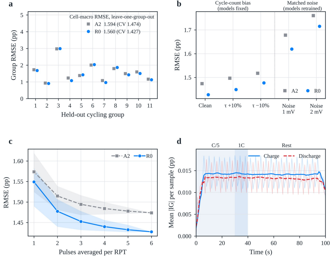
图 7 泛化性、稳健性与归因（复现实现）。 (a) 各循环工况组被留出时的组均 RMSE（留一工况组验证）；图例给出留一工况组验证下的电芯宏平均 RMSE，括号内为五折电芯互斥验证下的值。 (b) 测试循环数存在 \pm 10\% 偏差（模型固定）以及训练与测试数据中加入匹配高斯电压噪声（模型重新训练）时的 RMSE。 (c) RMSE 随每个 RPT 参与平均的脉冲数的变化；折线为全部工况组合的均值，色带为其范围。 (d) R0 在各波形采样点上的平均绝对积分梯度归因，实线为充电脉冲、虚线为放电脉冲，在测试记录、外层折与初始化种子间平均；阴影标示脉冲各区段。
