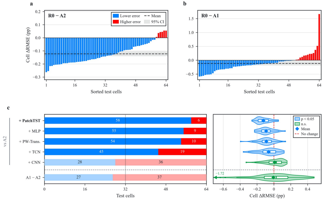
图 4 人工特征主干与波形补充的作用。(a) 64 个测试电芯的逐电芯 RMSE 差 R0 - A2（种子平均），按升序排列；蓝色柱表示 R0 误差更低，红色柱表示更高；虚线与灰带为平均差及其 95% 区间。(b) 同(a)，为 R0 - A1；最右侧一柱为电芯 3。(c) 左：MLP 主干加入各补充后误差降低（蓝）或升高（红）的电芯数，以及 A1 相对 A2 的情况（虚线下方）；浅色表示差异不显著。右：64 个配对差的小提琴图与箱线图（箱体为四分位距，线为中位数，须线延伸至 1.5 倍四分位距，菱形为均值）；超出坐标范围的一个值（A1 - A2，-1.72 个百分点，电芯 3）标于左侧边缘。
