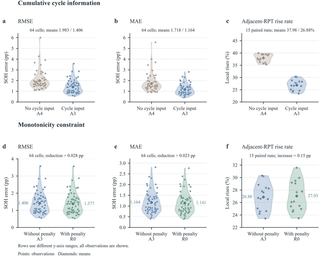
图6 累计循环信息与单调惩罚的作用。上排：A4（无循环数输入）与A3（有循环数输入）的比较，两者均不使用惩罚。下排：A3（无惩罚）与R0（有惩罚）的比较。（a, d）RMSE；（b, e）MAE；（c, f）相邻RPT间预测上升的比例。误差分布包含64个测试电芯（在初始化种子间平均）；上升率在同一电芯、名义SOC和脉冲方向内计算，涵盖15次运行。小提琴为限制在观测范围内的核密度；散点为观测值，菱形为均值。上下两排采用不同的纵轴范围。
