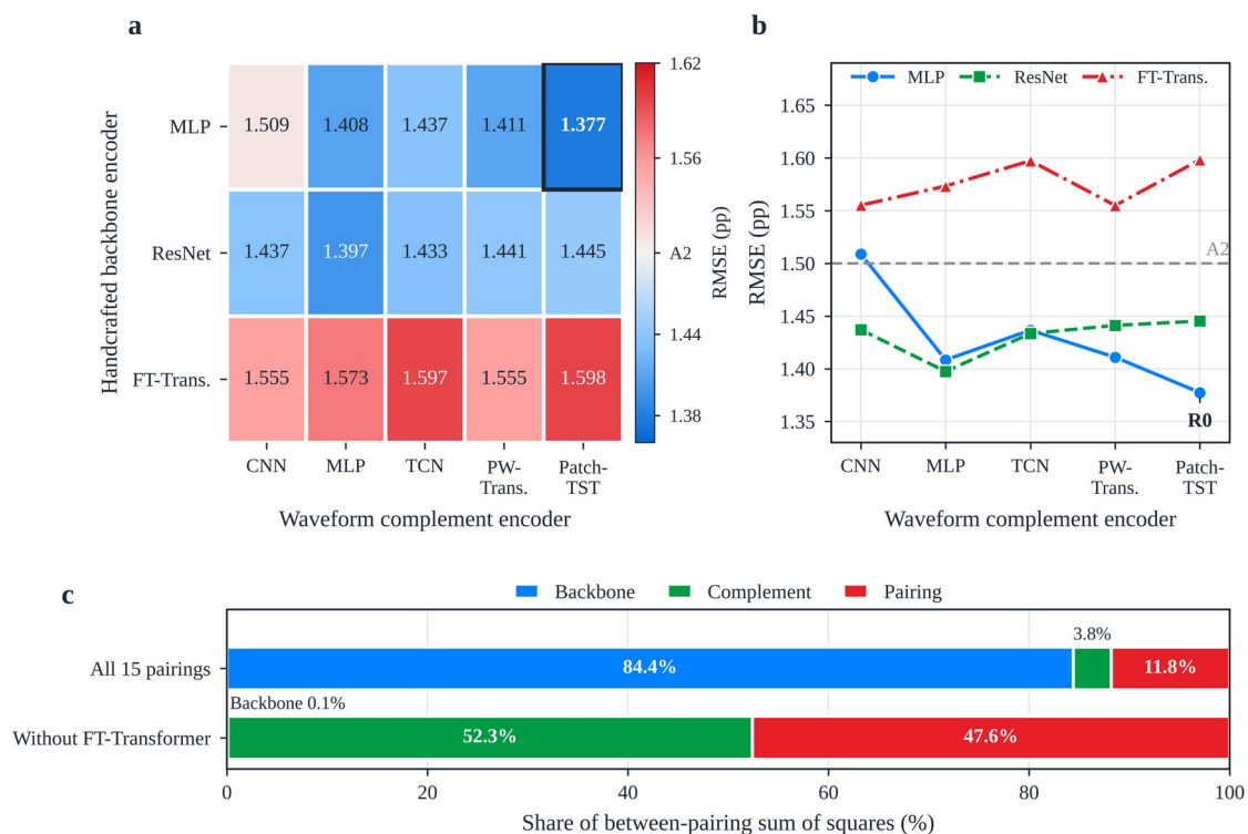
图 3 编码器比较矩阵的主效应与组合依赖。(a) 15 种组合的电芯宏平均 RMSE；发散色标以只含主干的模型 A2（1.500 个百分点）为中点，蓝色表示误差更低，红色表示更高；方框标出 R0。(b) 交互作用图；折线不平行
