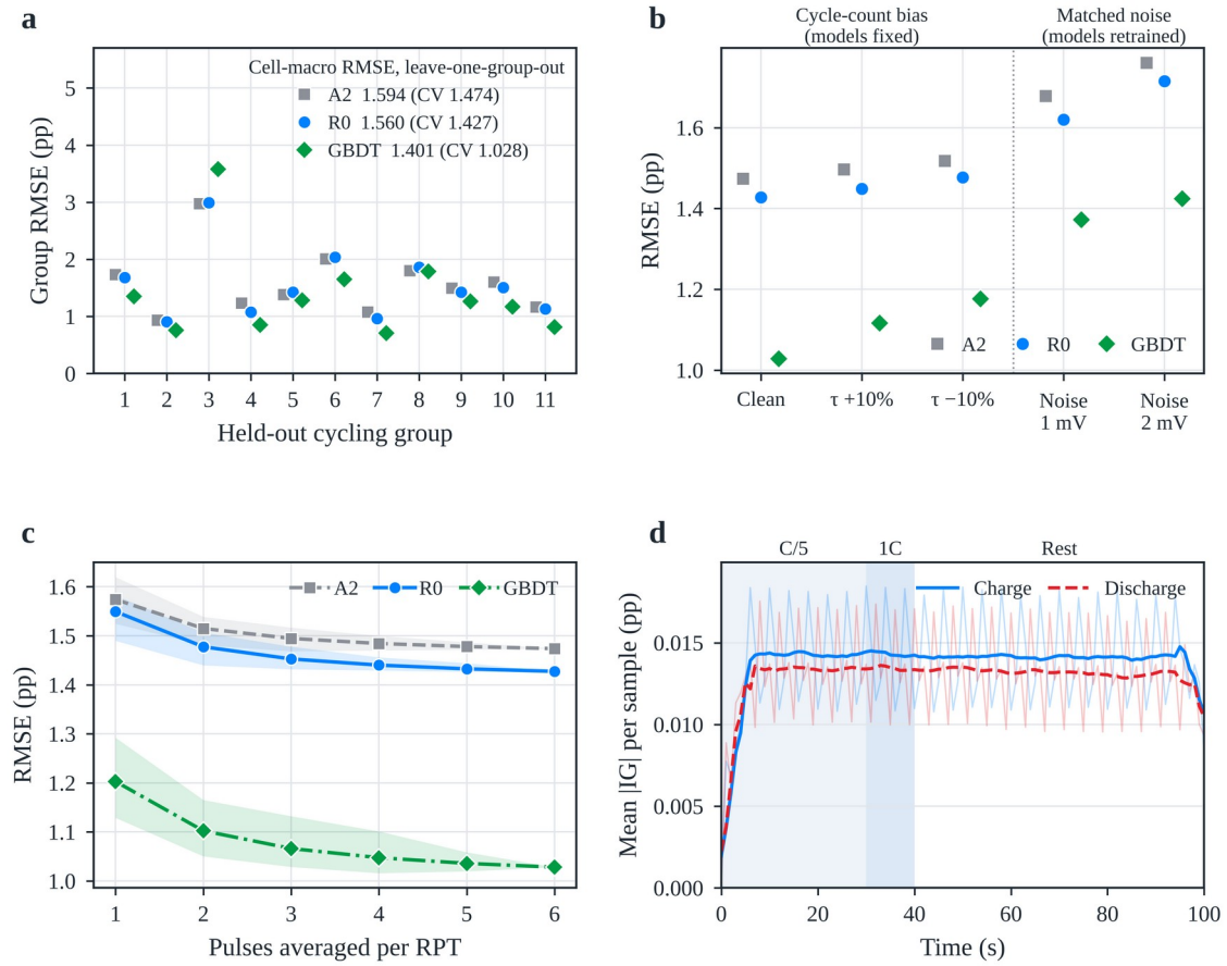
图 8 泛化性、稳健性与归因（复现实现）。(a) 各循环工况组被留出时的组均 RMSE（留一工况组验证）；图例给出留一工况组验证下的电芯宏平均 RMSE，括号内为五折电芯互斥验证下的值。(b) 测试循环数存在 \pm 10\% 偏差（模型固定）以及训练与测试数据中加入匹配高斯电压噪声（模型重新训练）时的 RMSE。(c) RMSE 随每个 RPT 参与平均的脉冲数的变化；折线为全部工况组合的均值，色带为其范围。(d) R0 在各波形采样点上的平均绝对积分梯度归因，实线为充电脉冲、虚线为放电脉冲，在测试记录、外层折与初始化种子间平均；阴影标示脉冲各区段。
