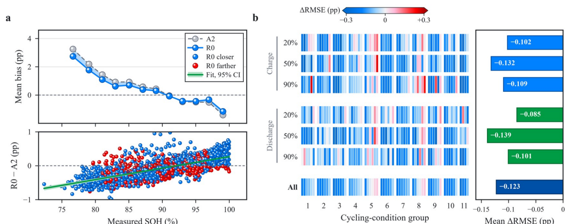
图 5 波形补充对偏差的修正及其在工况与电芯间的分布。(a) 上：按实测 SOH 每 2 个百分点分箱（低于 78% 的箱合并）的平均偏差（预测减真实值），灰色为 A2，蓝色为 R0；阴影表示被修正的偏差。下：2,823 个电芯-RPT 点上 R0 - A2 的预测改变量（蓝色表示更接近实测值，红色表示更远离），以及最小二乘拟合及其 95% bootstrap 区间带。预测均对种子和工况取平均。(b) 左：六个工况及全部记录上的逐电芯 R0 - A2 RMSE 差（电芯按循环工况组排列；超出 \pm 0.3 个百分点者颜色饱和）。右：各行的电芯宏平均差；所有 95% 区间均不含零。
