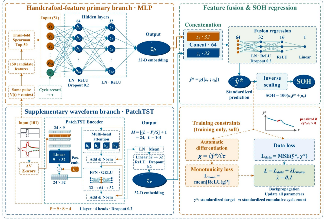
图 2 双分支 SOH 估计模型（R0 配置）。左上：人工特征主分支；训练折筛选的 50 项特征与标准化累计循环数 \tau 组成 51 维输入，经 MLP 编码为 32 维表征。左下：波形补充分支；101 点脉冲电压响应经首点作差与逐位置标准化后，划分为 24 个片段（片段长度 P=9 ，步长 S=4 ），由单层 PatchTST 编码为 32 维表征。右：两路表征拼接为 64 维，经回归得到标准化 SOH \hat{y}^* ，再经逆标准化输出。训练最小化均方误差与正偏导 \partial \hat{y}^*/\partial \tau 惩罚项之和（ \lambda=0.1 ）；该软约束仅在训练中起作用。
