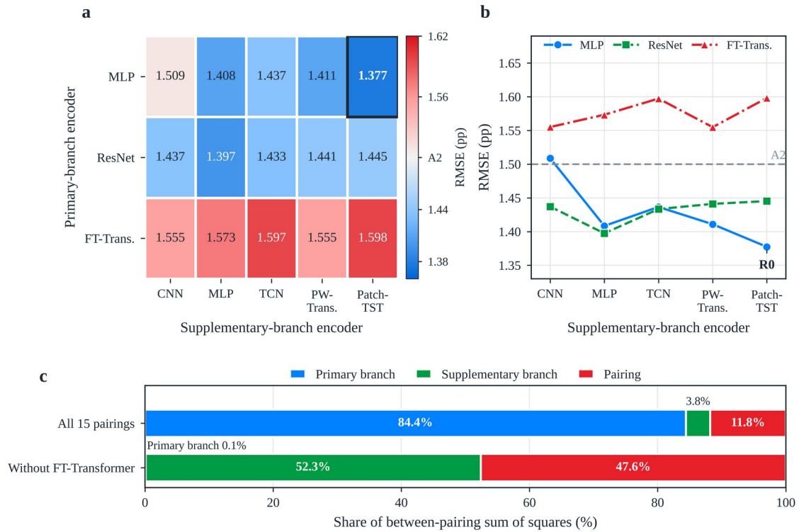
图 3 编码器比较矩阵的主效应与组合依赖。(a) 15 种组合的电芯宏平均 RMSE；发散色标以只含主分支的模型 A2（1.500 个百分点）为中点，蓝色表示误差更低，红色表示更高；方框标出 R0。(b) 交互作用图；折线不平行表示存在组合依赖；虚线为 A2。(c) 主分支编码器、补充分支编码器及组合依赖在组间平方和中所占的比例：全部 15 种组合（95% 区间：73.1~90.2%、1.9~8.1%、7.3~20.2%）及去掉 FT-Transformer 后（0.0~4.6%、40.4~65.0%、34.1~58.4%），区间来自 5,000 次折分层电芯 bootstrap。数值为 225 次训练的种子平均电芯指标。
