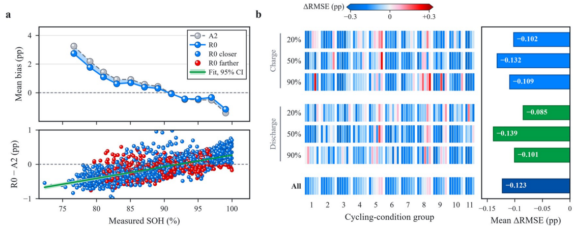
图5 波形补充分支对偏差的修正及其在工况与电芯间的分布。(a) 上：按实测 SOH 每 2 个百分点分箱（低于 78% 的箱合并）的平均偏差（预测减真实值），灰色为 A2，蓝色为 R0；阴影表示被修正的偏差。下：2,823 个电芯-RPT 点上 R0 - A2 的预测改变量（蓝色表示更接近实测值，红色表示更远离），以及最小二乘拟合及其 95% bootstrap 区间带。预测均对种子和工况取平均。(b) 左：六个工况及全部记录上的逐电芯 R0 - A2 RMSE 差（电芯按循环工况组排列；超出 \pm 0.3 个百分点者颜色饱和）。右：各行的电芯宏平均差；所有 95% 区间均不含零。
