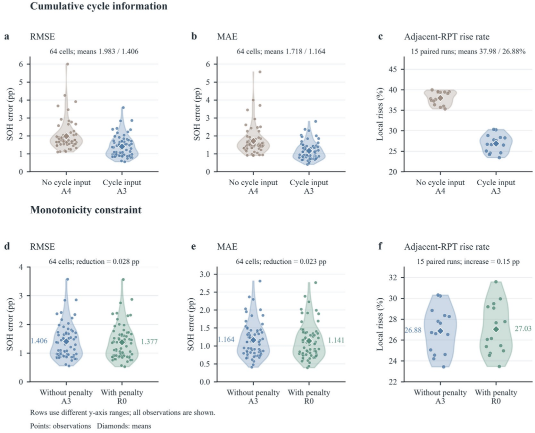
图 6 累计循环信息与单调惩罚的作用。上排：A4（无循环数输入）与 A3（有循环数输入）的比较，两者均不使用惩罚。下排：A3（无惩罚）与 R0（有惩罚）的比较。（a, d）RMSE；（b, e）MAE；（c, f）相邻 RPT 间预测上升的比例。误差分布包含 64 个测试电芯（在初始化种子间平均）；上升率在同一电芯、名义 SOC 和脉冲方向内计算，涵盖 15 次运行。小提琴为限制在观测范围内的核密度；散点为观测值，菱形为均值。上下两排采用不同的纵轴范围。
