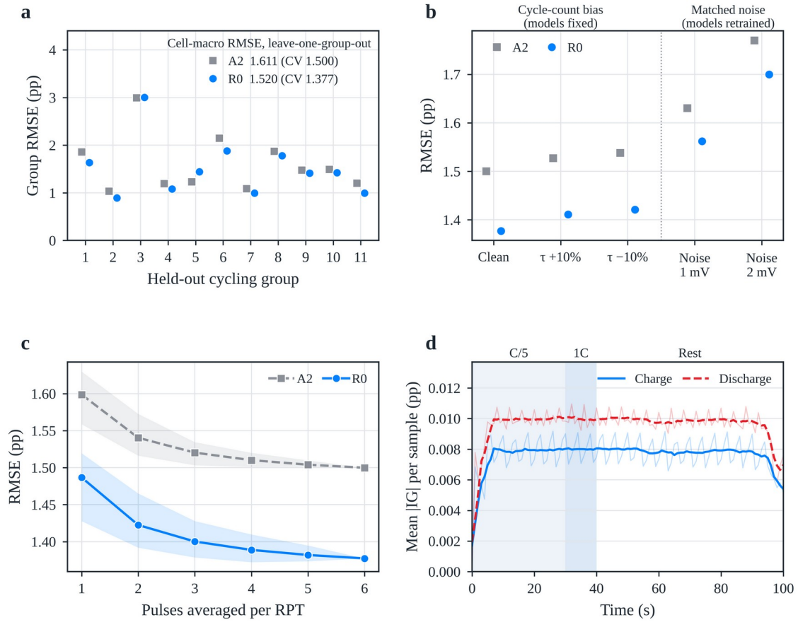
图7 泛化性、稳健性与归因。(a) 各循环工况组被留出时的组均 RMSE（留一工况组验证）；图例给出留一工况组验证下的电芯宏平均 RMSE，括号内为五折电芯互斥验证下的值。(b) 测试循环数存在 \pm 10\% 偏差（模型固定）以及训练与测试数据中加入匹配高斯电压噪声（模型重新训练）时的 RMSE。(c) RMSE 随每个 RPT 参与平均的脉冲数的变化；折线为全部工况组合的均值，色带为其范围。(d) R0 在各波形采样点上的平均绝对积分梯度归因，实线为充电脉冲、虚线为放电脉冲，在测试记录、外层折与初始化种子间平均；阴影标示脉冲各区间。
