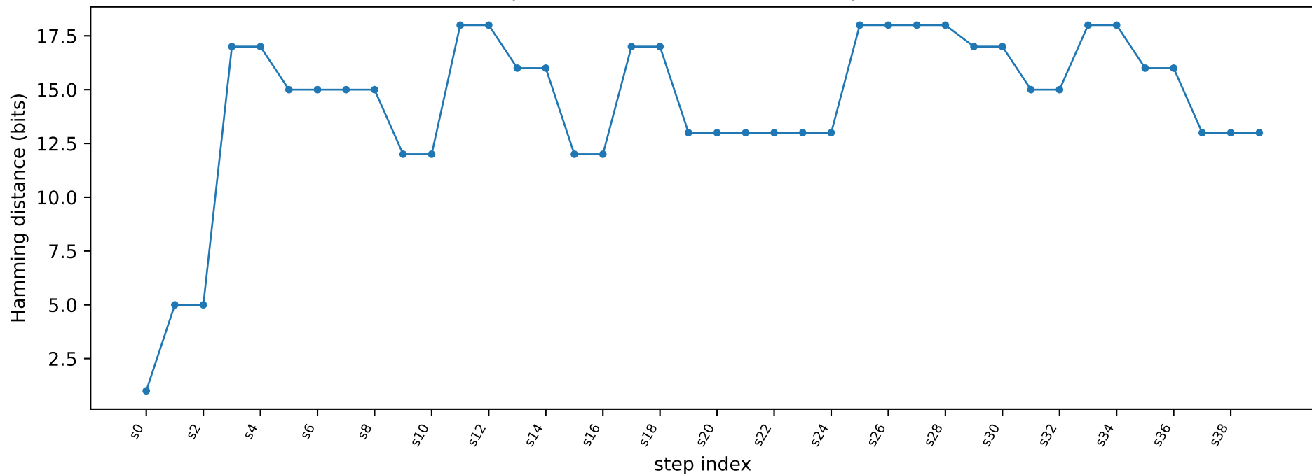
Q1 part b no shiftrows (P vs P', key fixed)
