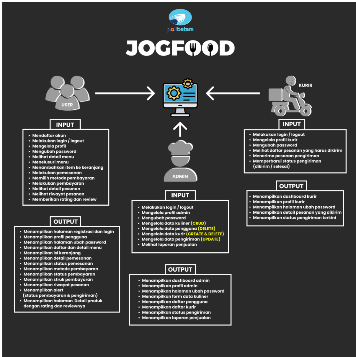
Gambar 1 Desain Umum Aplikasi Jogfood
