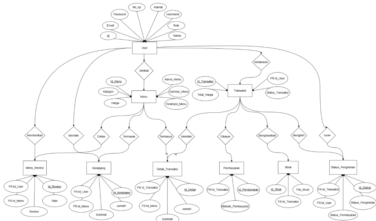
Gambar 3 ER Diagram Aplikasi Jogfood
