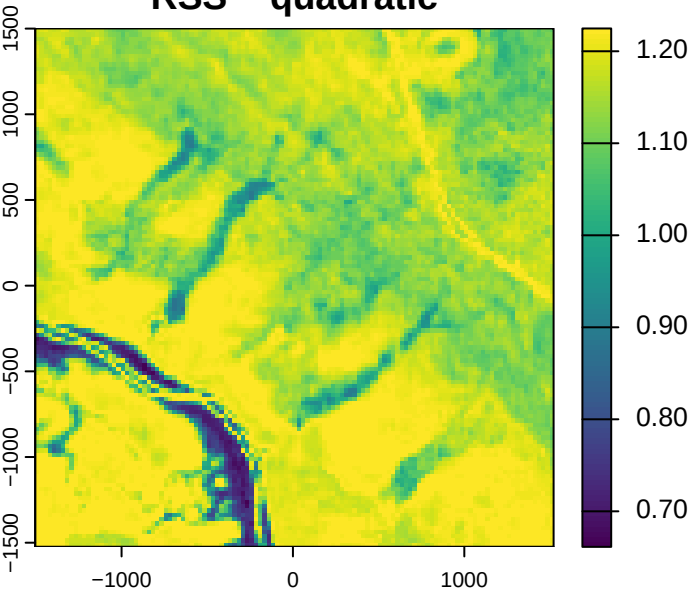
RSS - quadratic
