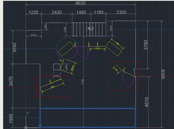
실측 치수를 반영한 무대 도면
