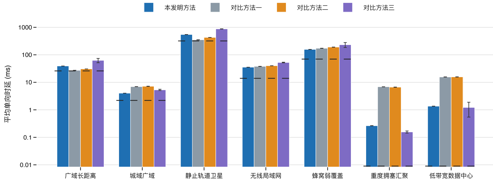
平均单向前向时延（短划线为基线传播时延）
