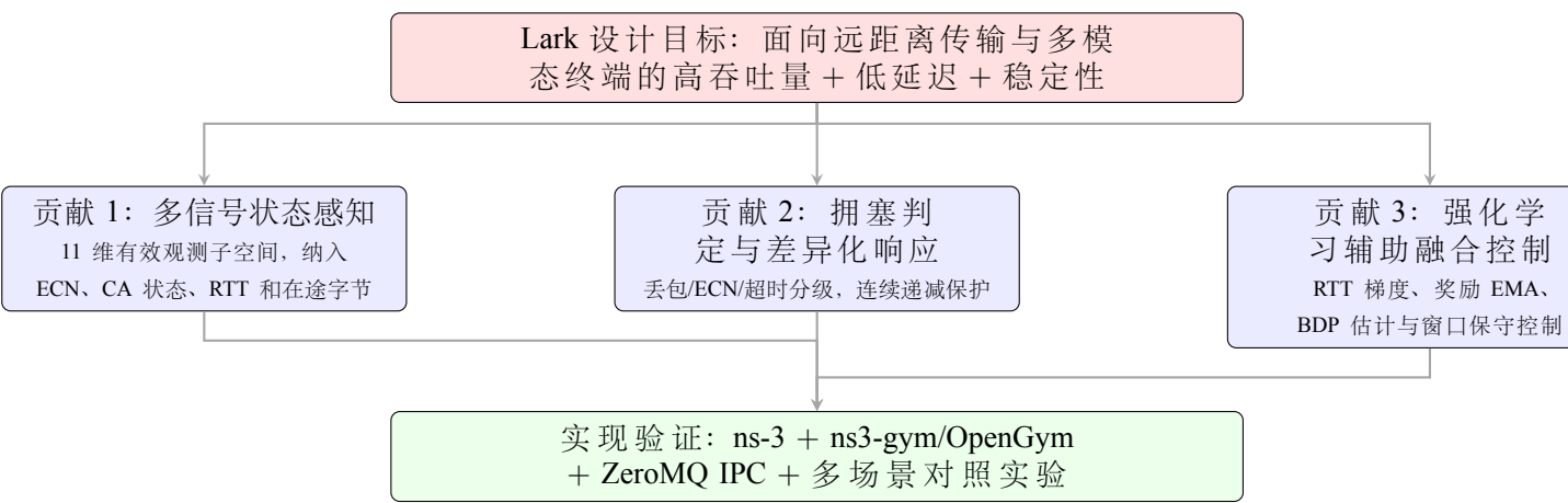
图 1.1 Lark 算法核心贡献概览
