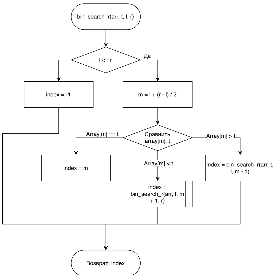
Рисунок 2.4 — Схема рекурсивного алгоритма бинарного поиска
