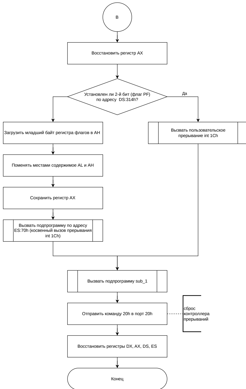
Рисунок 4 – Схема алгоритма работы обработчика прерывания INT 8h
