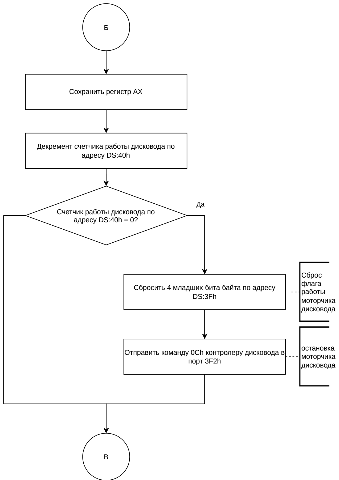
Рисунок 3 – Схема алгоритма работы обработчика прерывания INT 8h
