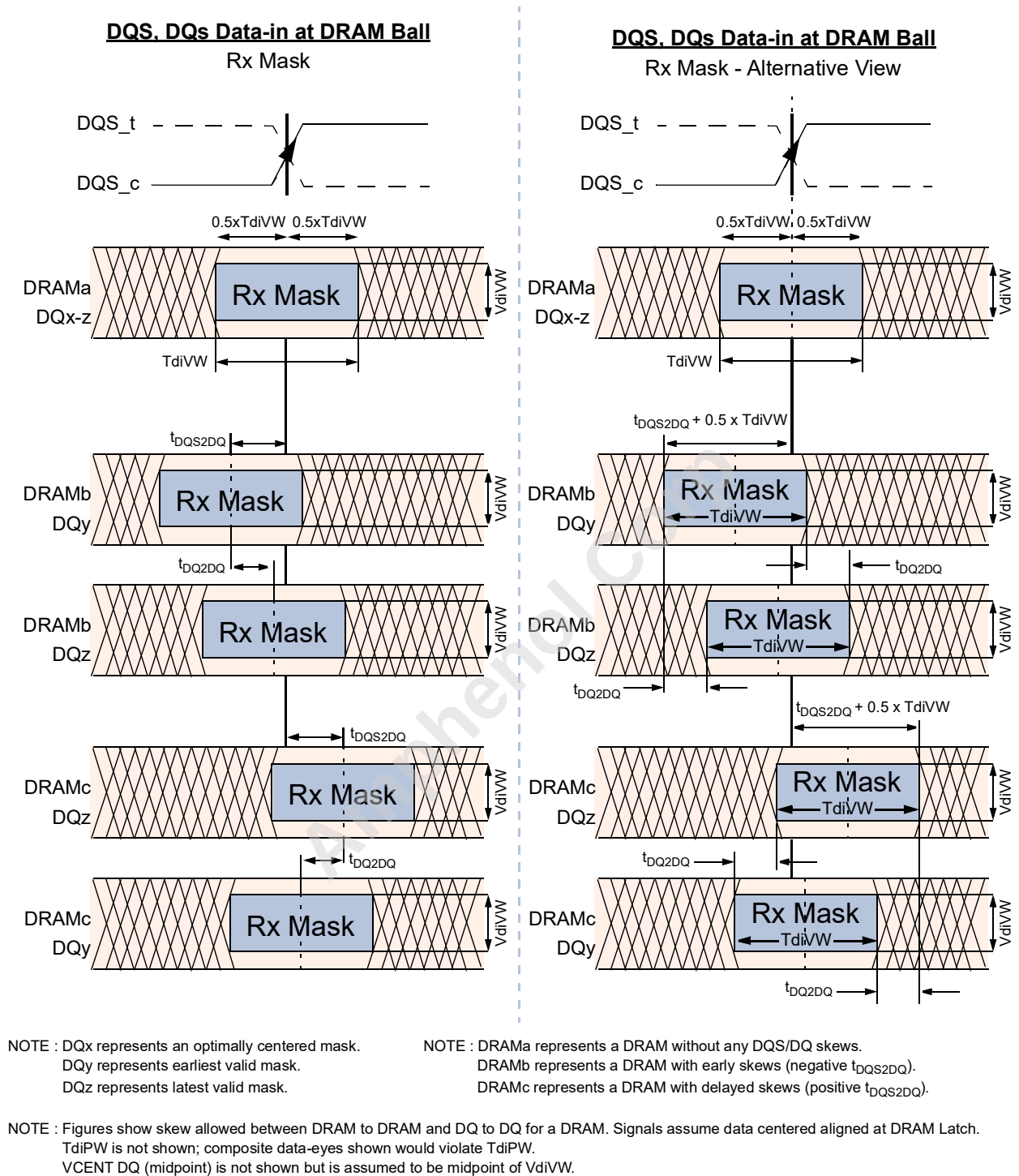
Figure 230 — DQS to DQ and DQ to DQ Timings at DRAM Balls
