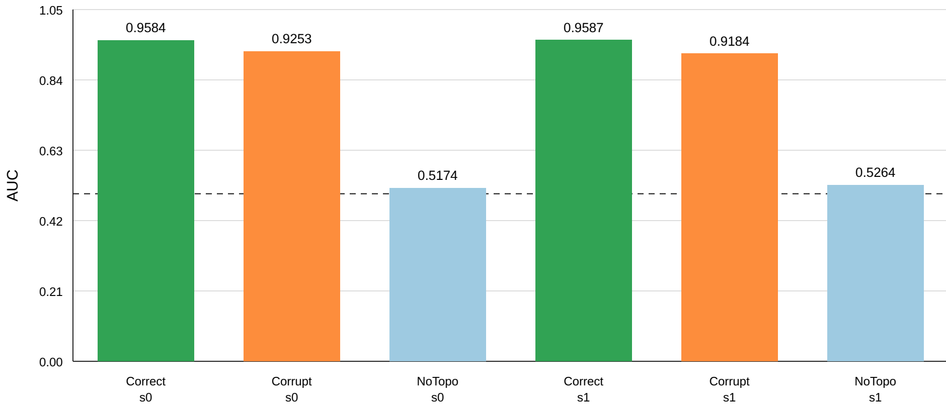
Dialga-128 r4 D2: 同一检查点替换结构说明书 (2048/class)
