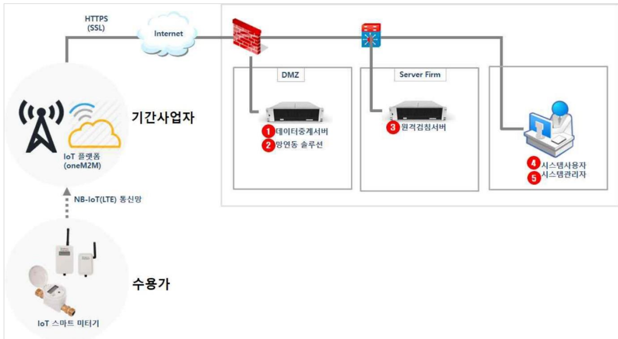
그림 1 원격검침 시스템
