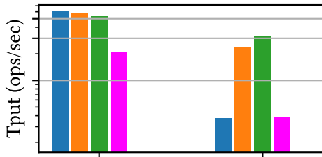
YCSB B
