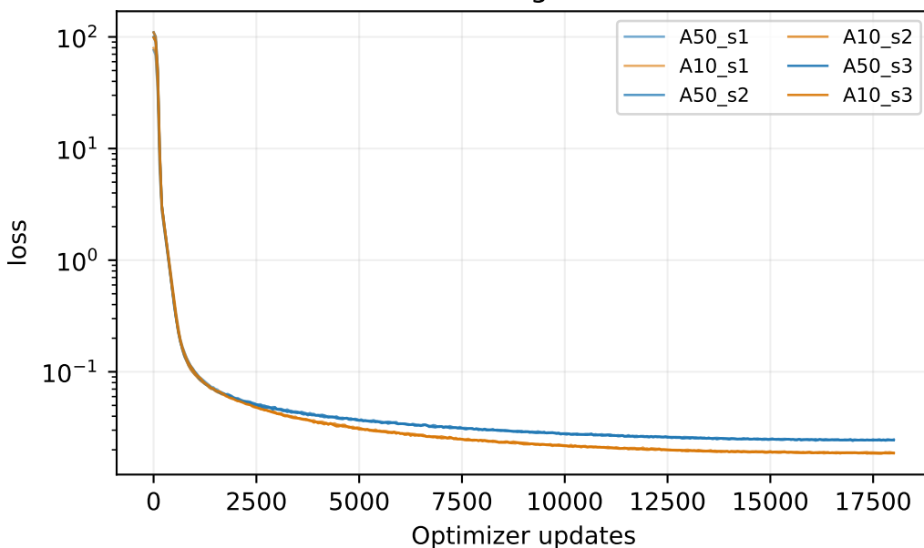
Training kl
