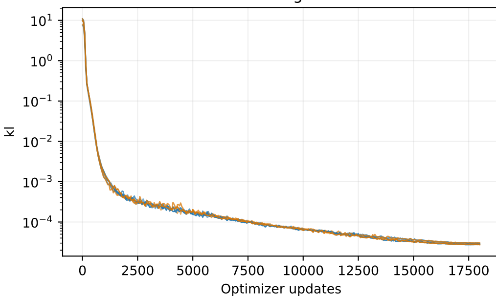
Training kl
