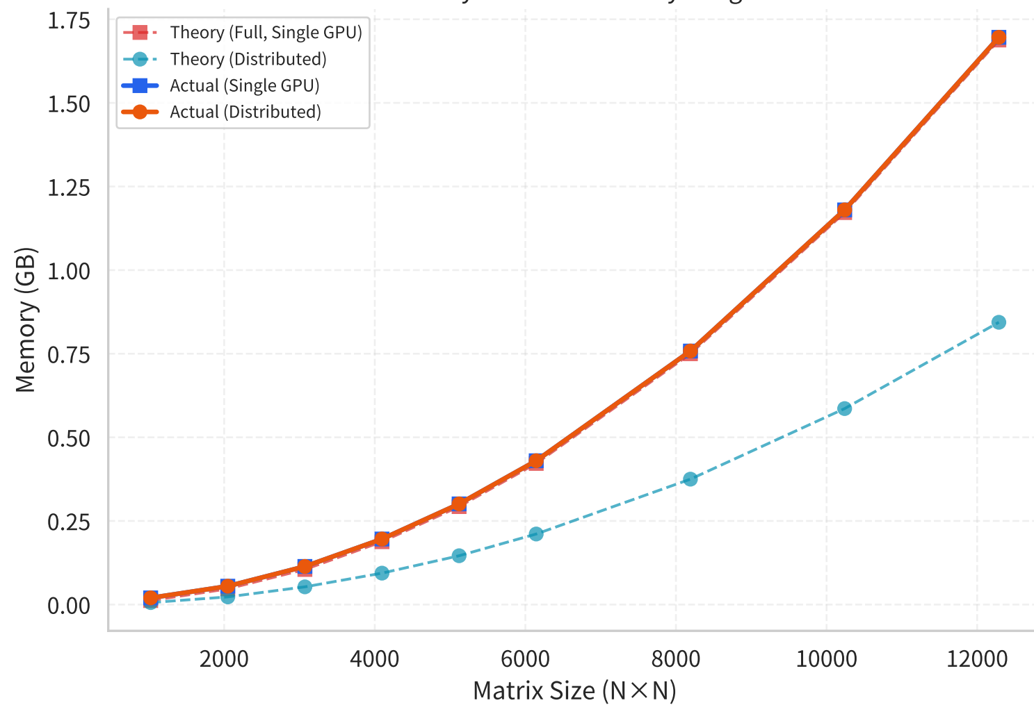
Theory vs Actual Memory Usage
