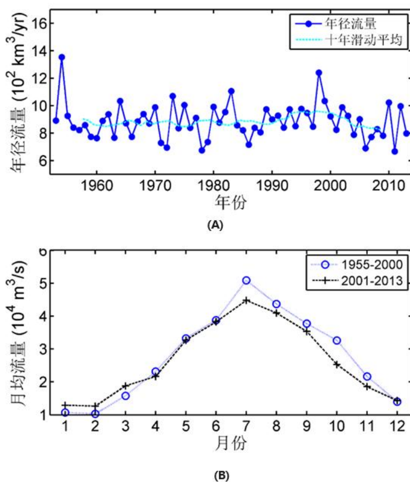
图 2-6 长江径流量年际变化(A)及(B)年内分布
