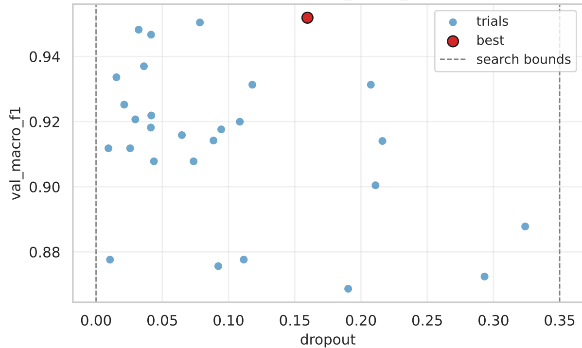
dropout vs val_macro_f1
