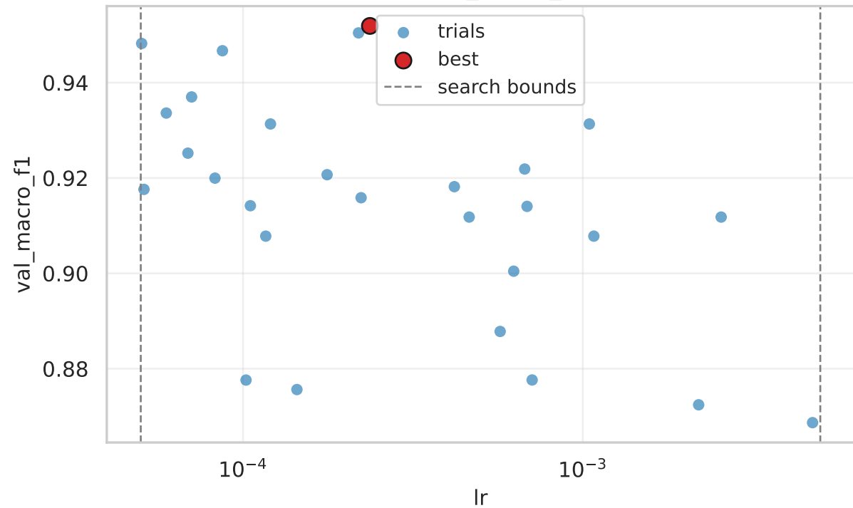
lr vs val_macro_f1
