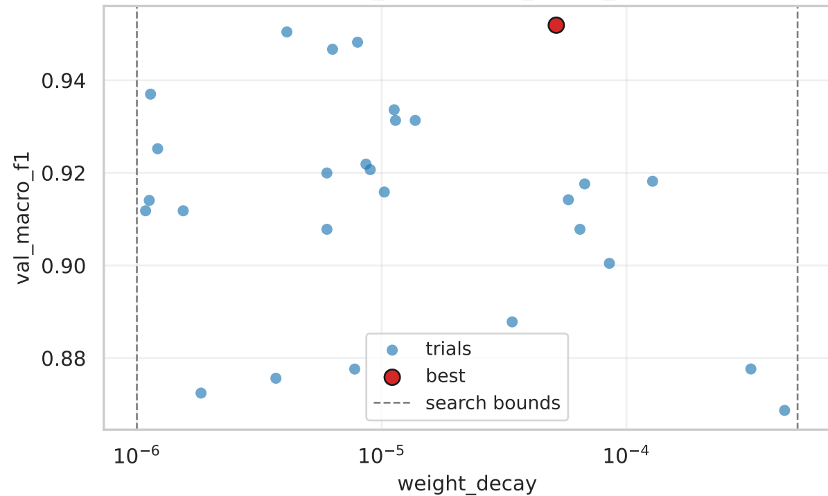
weight_decay vs val_macro_f1
