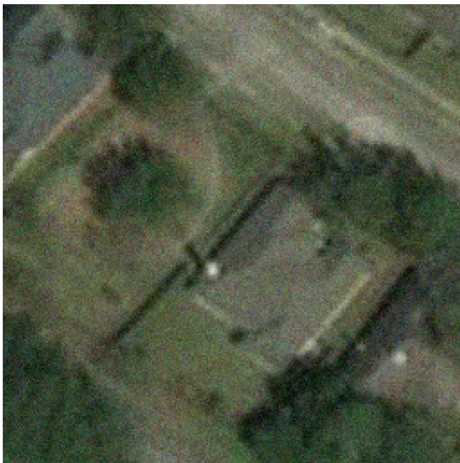
test/no_damage,-95.632351_29.767795.jpeg
