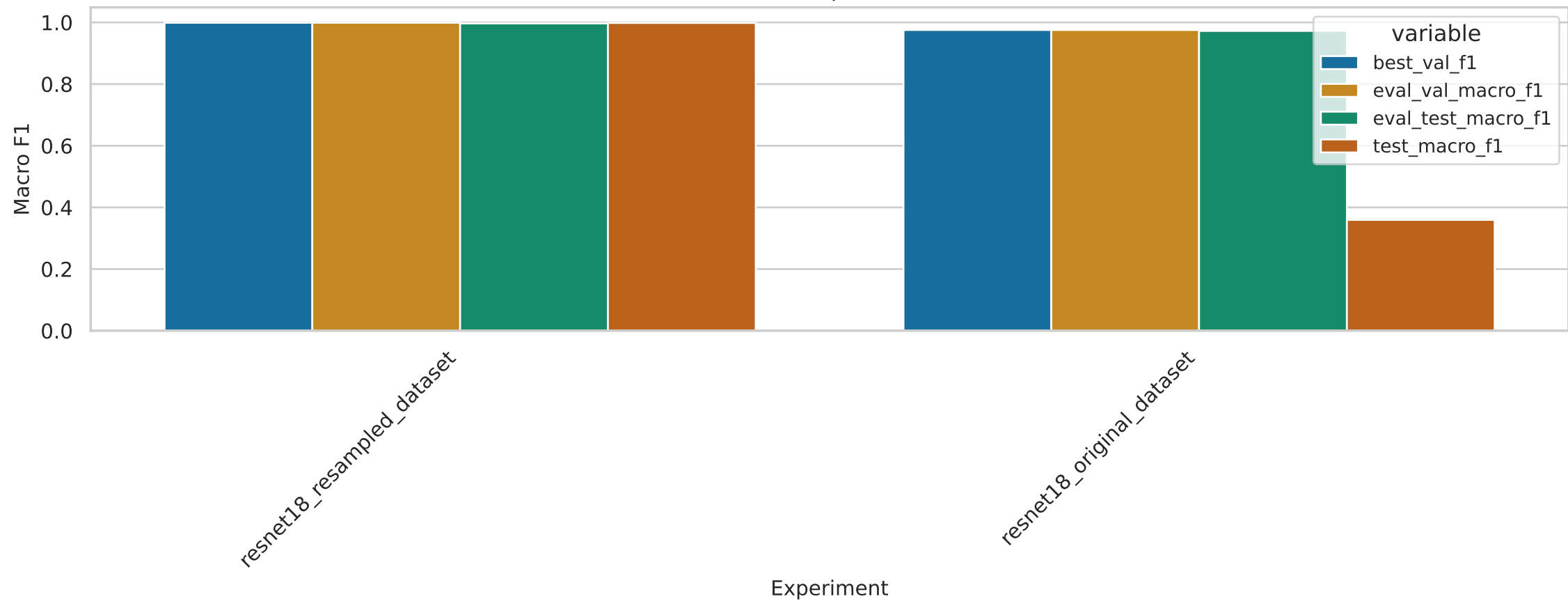
F1 Comparison
