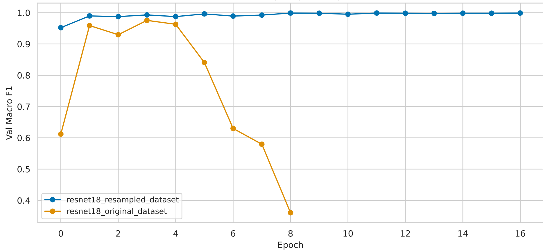
Validation F1 per Epoch (top runs)
