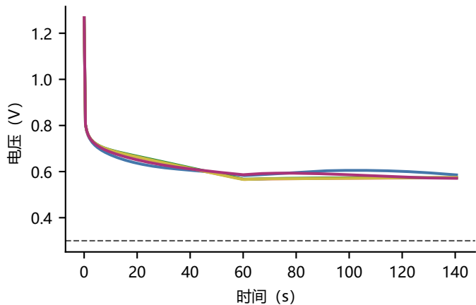
问题4：完全冷却，动态功率控制（启动时间折中）
