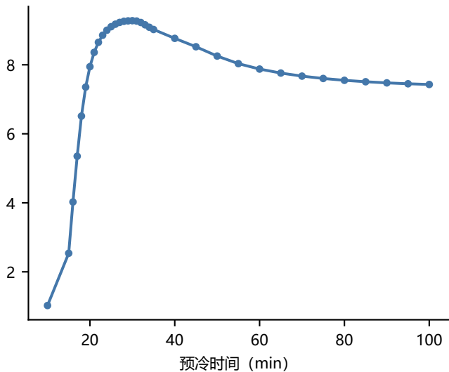
启动过程最大片间温差 (K)
