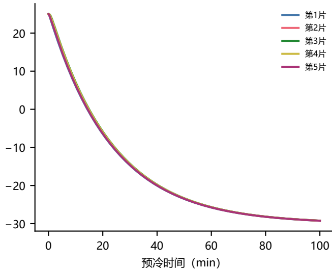
单片平均温度 (°C)
