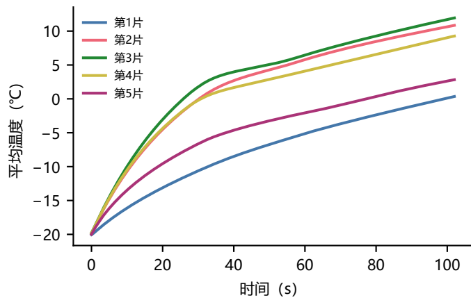
问题4：预冷40 min，动态功率控制（启动时间折中）
