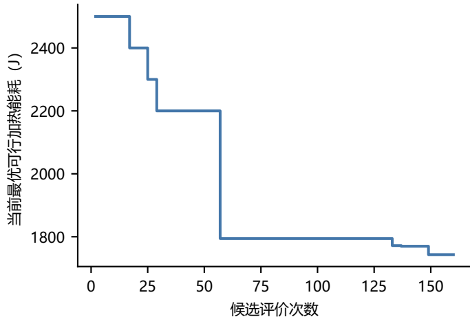
问题3：恒功率协同加热搜索 原300 s时域搜索
