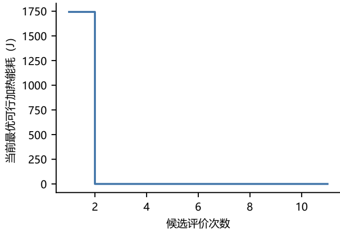
问题4: 预冷40 min恒功率重优化 原300 s时域搜索
