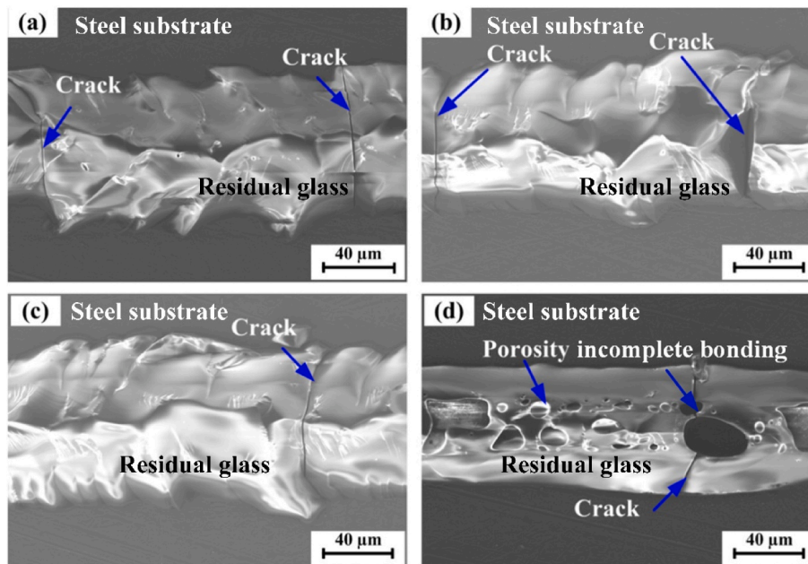
Fig. 4. Weld fracture at different pulse power levels: (a) 8 W; (b) 12 W; (c) 16 W; (d) 20 W.
